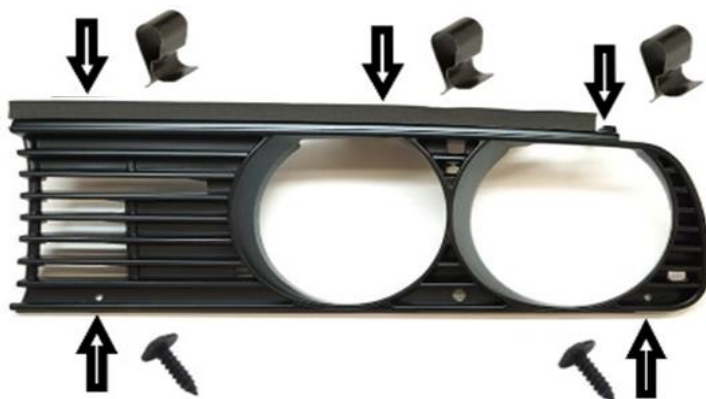
Photo 2 (Détails du montage de la grille du phare BMW E30)
