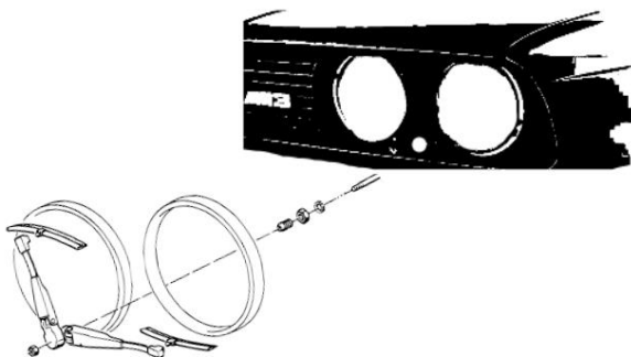
Photo 6 (Installation de l'essuie-glace)
